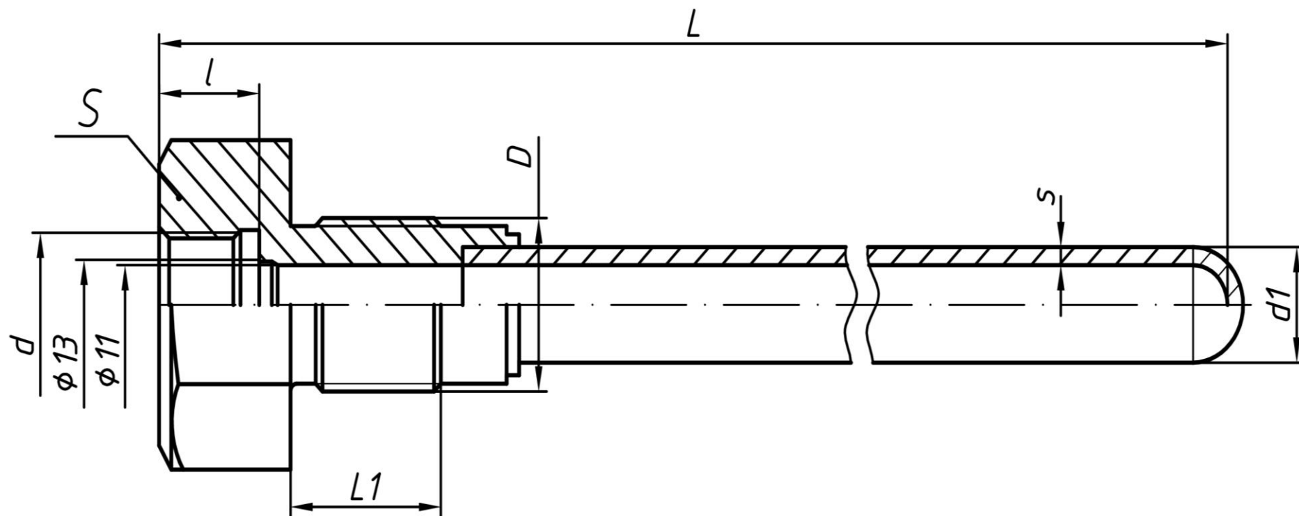
Рисунок 7 – Гильза ГЗШ - 3
