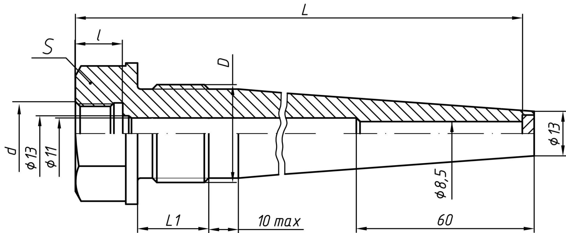
Рисунок 5 – Гильза ГЗШ - 1
