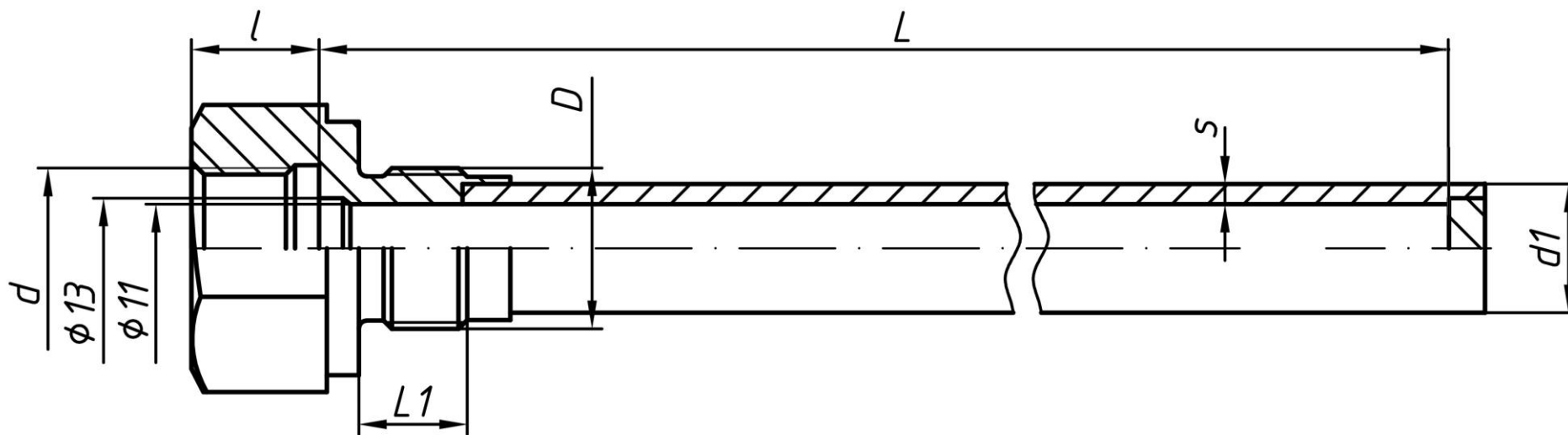
Рисунок 4 – Гильза ГЗШ - 4
