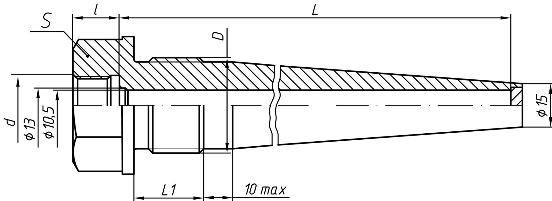
Рисунок 2 – Гильза ГЗШ-2
