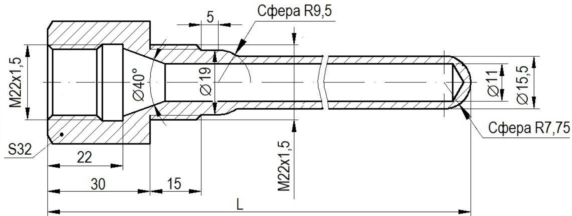
Рисунок 13 – Гильза ГЗШ-1172 (ЮВМА.408721.158) (для датчиков температуры с подвижным штуцером)
