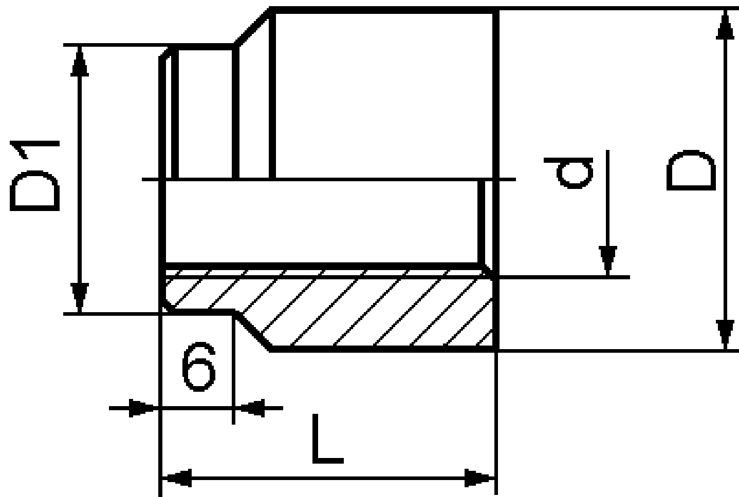
Рисунок 2 – Бобышка тип 2 (под неподвижный штуцер)
