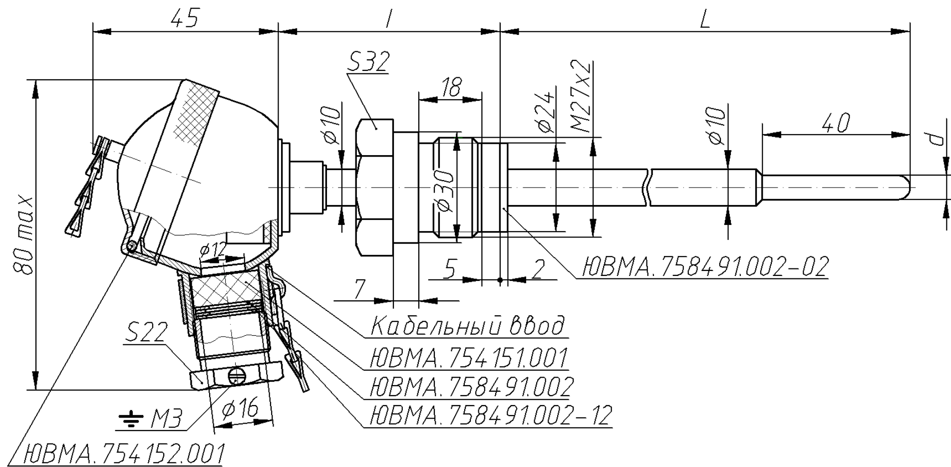
Рисунок В.2 – Штуцер неподвижный
