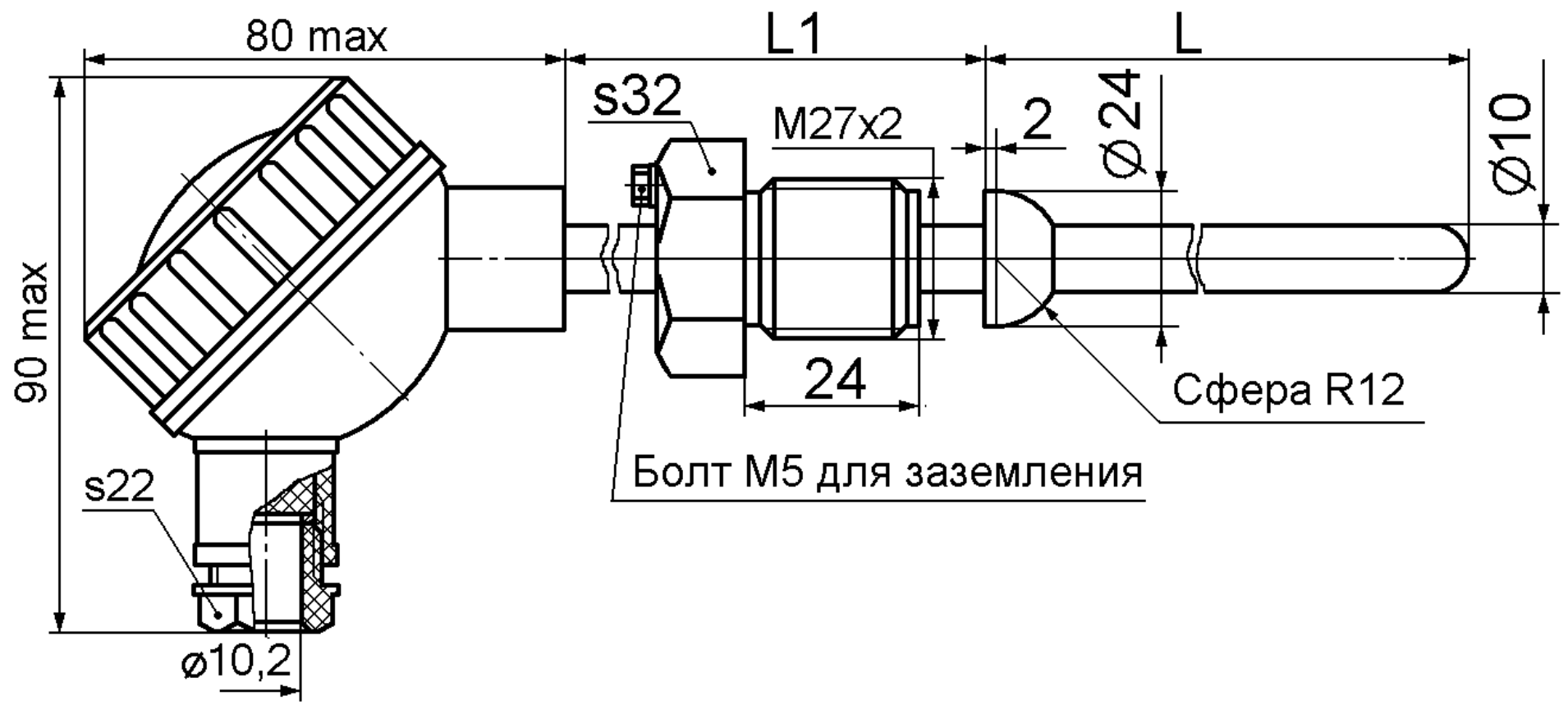
Рисунок В.2 – Штуцер подвижный
