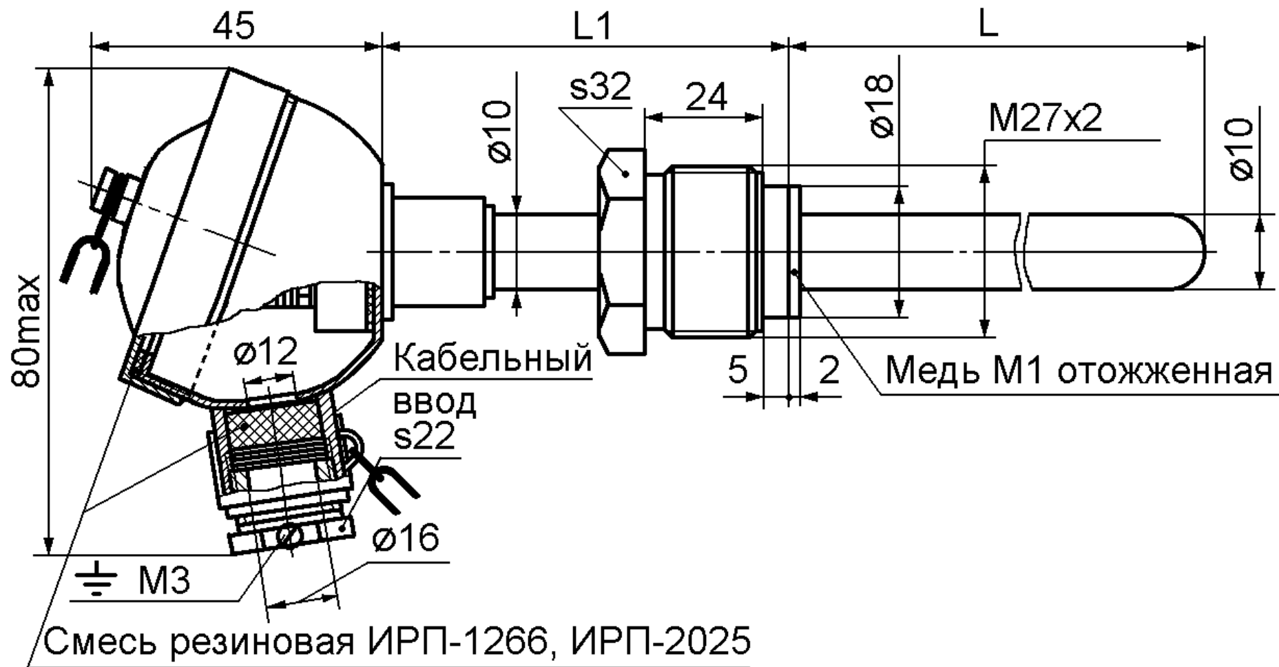
Рисунок Г.3 – Штуцер подвижный
